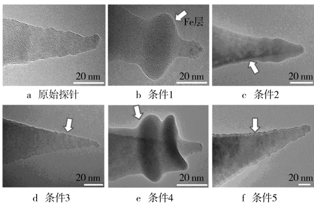
图 1 不同实验条件下的探针前端 TEM 图
