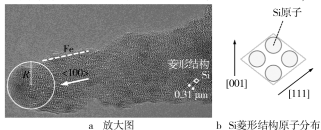
图 2 探针针尖的前端放大图及 Si 的菱形结构原子分布示意图
