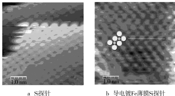
图 3 利用 Si 探针和导电镀 Fe 薄膜 Si 探针扫描 NaCl(001) 表面 Fig. 3 The AFM topography of NaCl (001) surface using Si probe without and with Fe film coating
